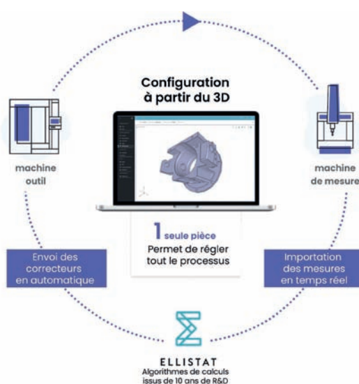
► Aperçu de l'APC en boucle fermée
